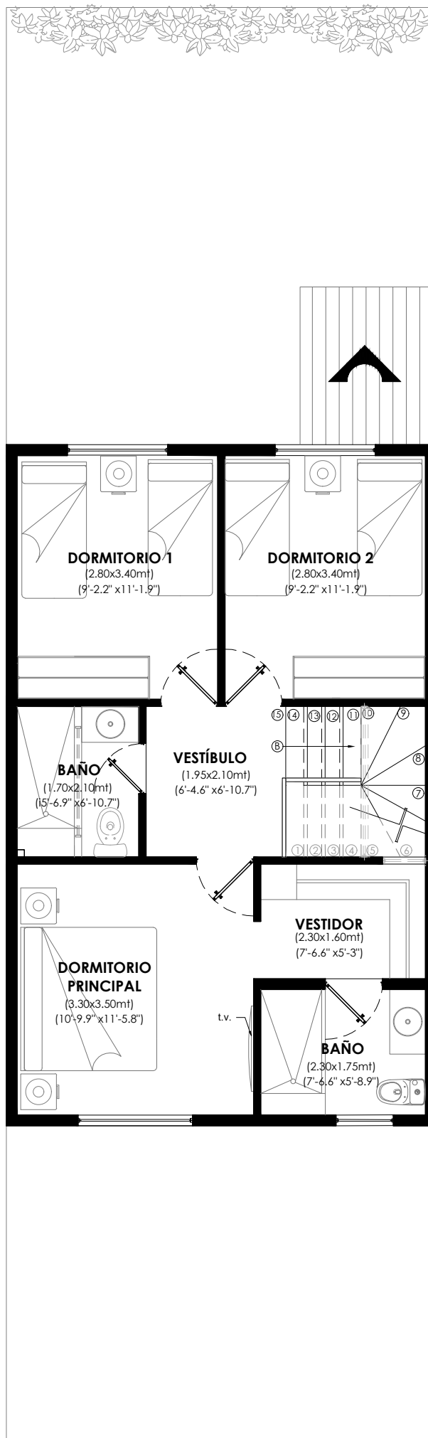
SEGUNDO NIVEL
